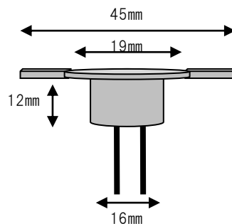
「ディスク型サーモスタットの場合」
