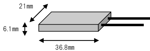
「平型サーモスタットの場合」
